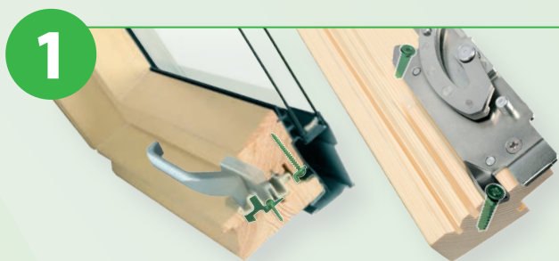
1 Антивандальна система «topSafe»
